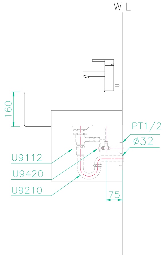
(설치구 가공도)
