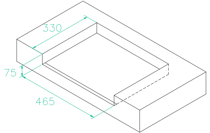
(설치구 가공도)
